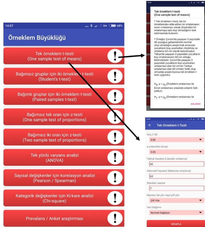
Şekil 3. Mobil uygulama kullanım örneği; “tek örneklem t-test” için örneklem büyüklüğü hesaplama bölümü ekran görüntüsü
