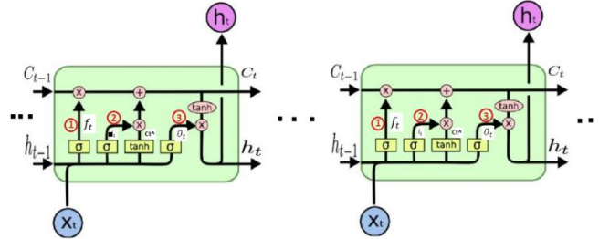
Şekil 1. LSTM Algoritma Mimarisi
