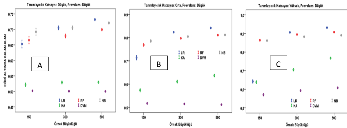
Şekil 2. Düşük, orta ve yüksek tanımlayıcılık katsayısı, yüksek prevalans senaryolarında üç örnek büyüklüğü için doğruluk değerinin her bir sınıflama yöntemi için ortalama ve % 95 güven aralıkları
