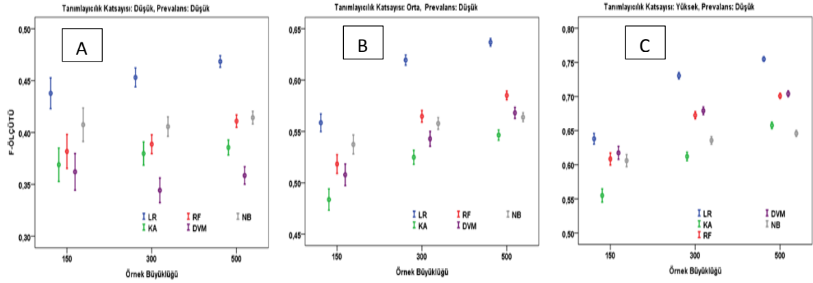
Şekil 5. Düşük, orta ve yüksek tanımlayıcılık katsayısı, düşük prevalans senaryolarında üç örnek büyüklüğü için F-ölçütü değerinin her bir sınıflama yöntemi için ortalama ve % 95 güven aralıkları
