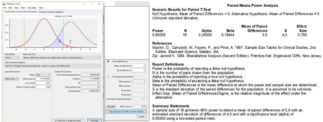
Şekil 7. G*Power ve PASS paketleri “eşleştirilmiş t-test” için örneklem büyüklüğü raporu
