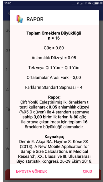
Şekil 6. Mobil uygulama “eşleştirilmiş t-test” için örneklem büyüklüğü raporu
