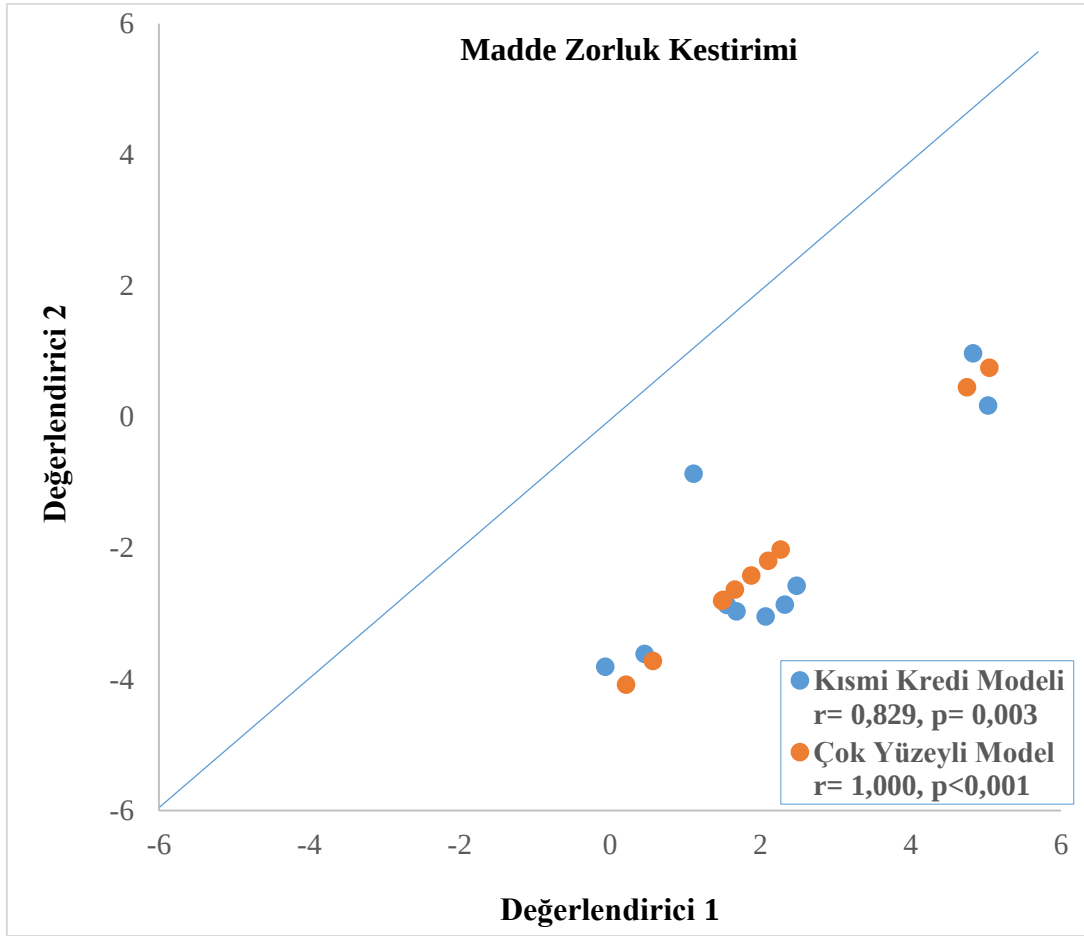
Şekil 3. İki değerlendiricinin tutumları birbirinden farklı olduğu durumda oluşturulan veri setinde kısmi kredi modeli ile çok yüzeyli Rasch modeli arasındaki ilişki
