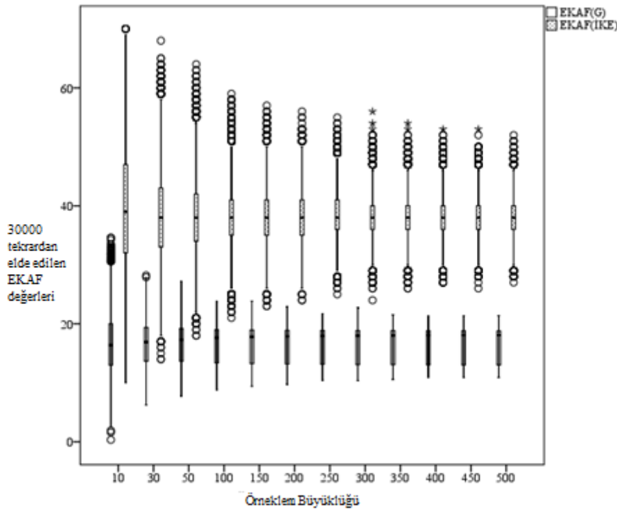
Şekil 3. Her bir örneklem büyüklüğü kategorisine ilişkin 30000 tekrardan elde edilen sonuçların özeti
