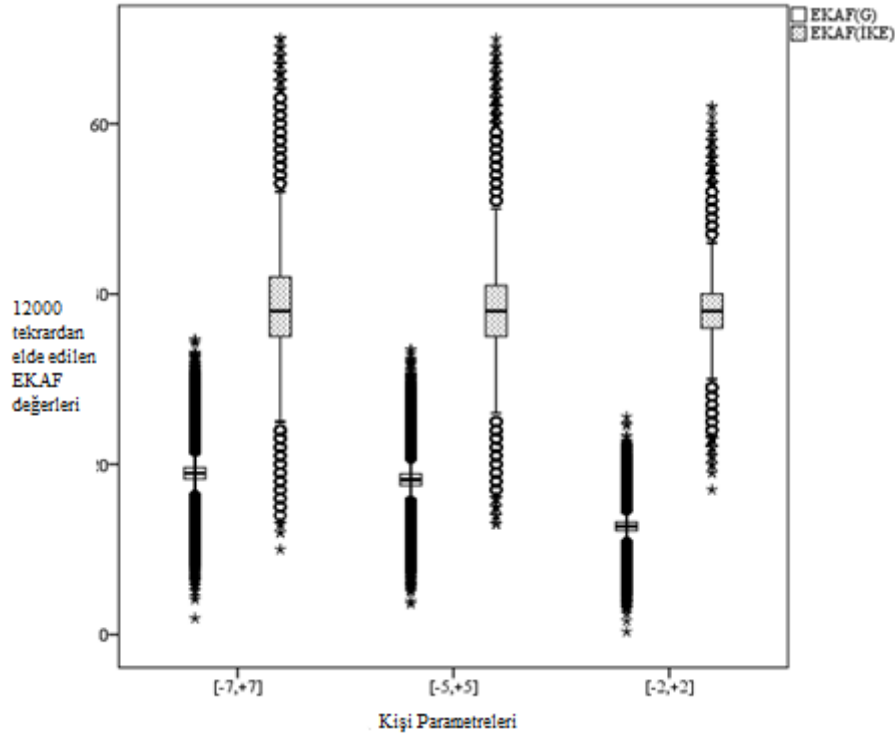
Şekil 2. Her bir kişi parametre kategorisine ilişkin 12000 tekrardan elde edilen sonuçların özeti
