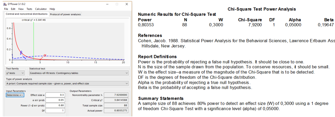
Şekil 9. G*Power ve PASS paketleri “ki-kare test” için örneklem büyüklüğü raporu
