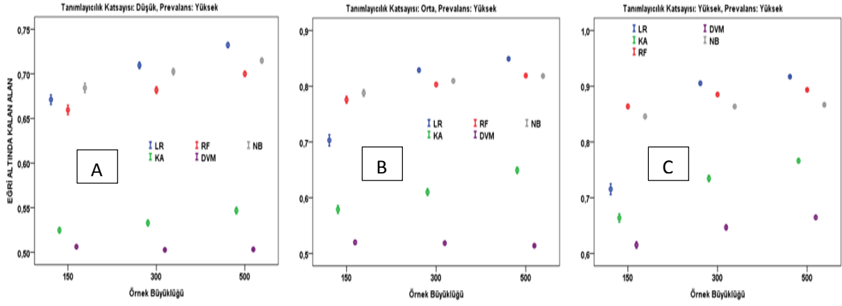
Şekil 4. Düşük, orta ve yüksek tanımlayıcılık katsayısı, yüksek prevalans senaryolarında üç örnek büyüklüğü için EAKA değerinin her bir sınıflama yöntemi için ortalama ve % 95 güven aralıkları
