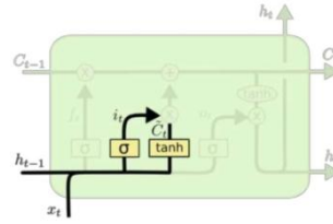
Şekil 3. Giriş Kapısı
