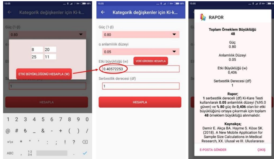
Şekil 10. Mobil uygulama “ki-kare test” için etki büyüklüğü hesaplaması ve örneklem büyüklüğü raporu
