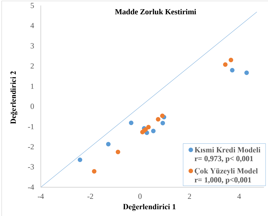
Şekil 1. Orijinal veri setinde kısmi kredi modeli ile çok yüzeyle Rasch modeli madde zorluk kestirimleri arasındaki ilişki
