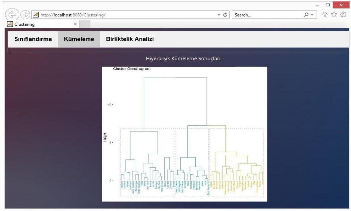
Şekil 1. Üç kümeye ait dendrogram yapısı
