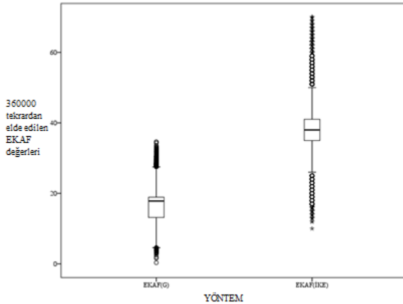
Şekil 1. 360000 tekrardan elde edilen sonuçların özeti
