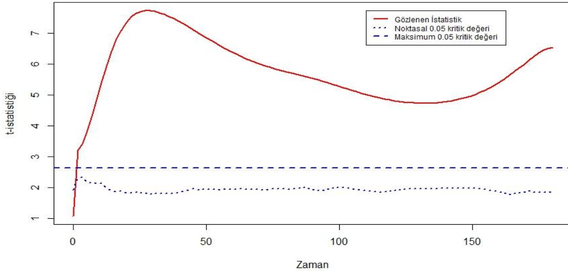
Şekil 4. Tedavi grupları arasındaki farka ilişkin permütasyon testi
