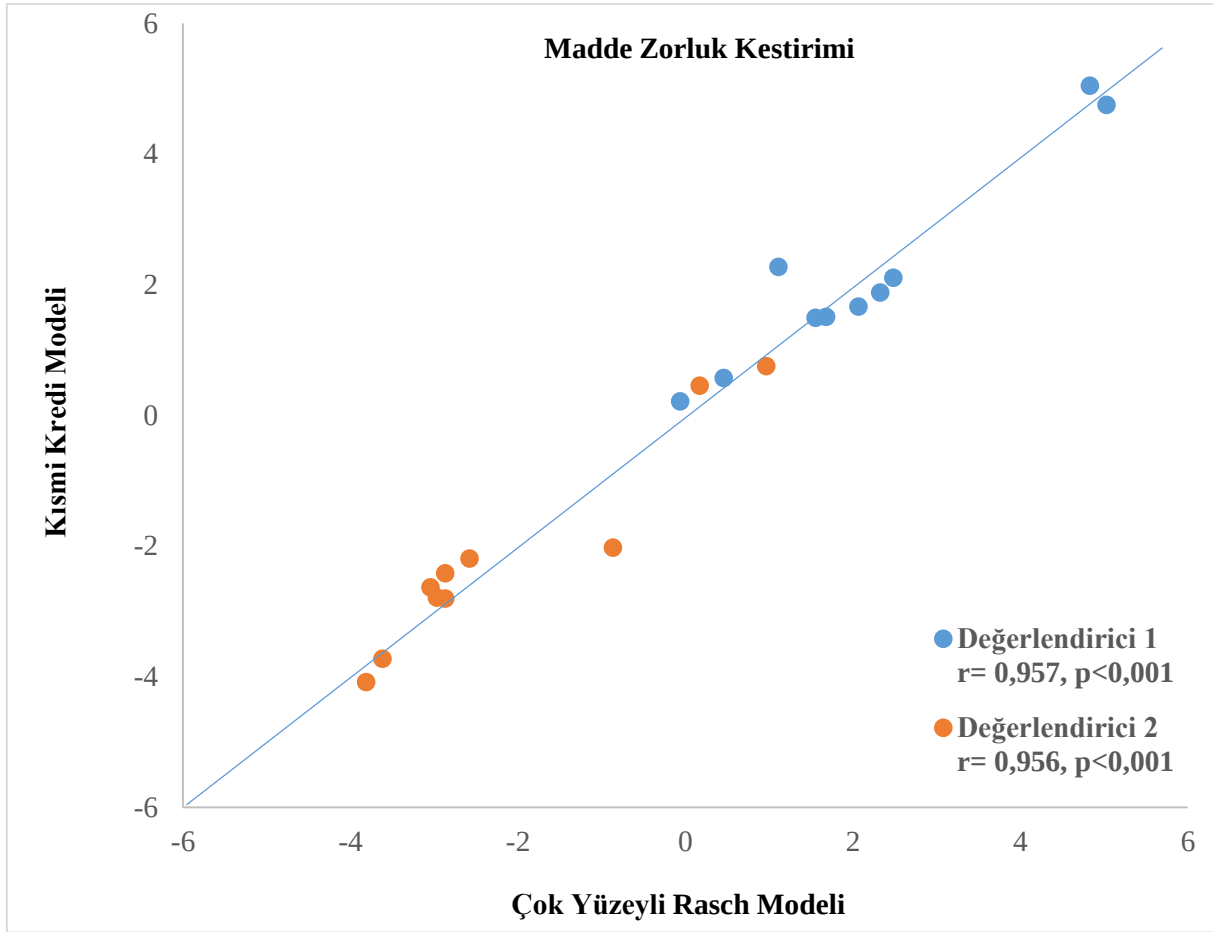
Şekil 4. İki değerlendiricinin tutumları birbirinden farklı olduğu durumda oluşturulan veri setinde değerlendiriciler için kısmi kredi modeli ile çok yüzeyli Rasch modeli arasındaki ilişki
