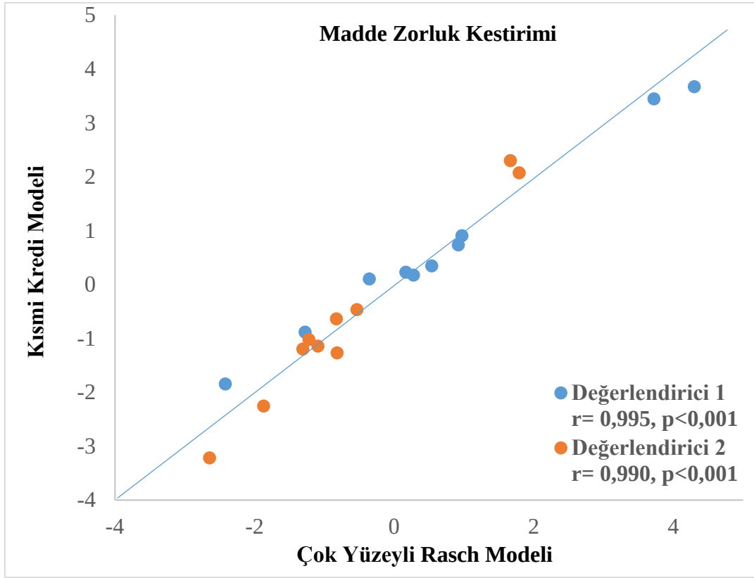
Şekil 2. Orijinal veri setinde değerlendiriciler için kısmi kredi modeli ile çok yüzeyle Rasch modeli madde zorluk kestirimleri arasındaki ilişki
