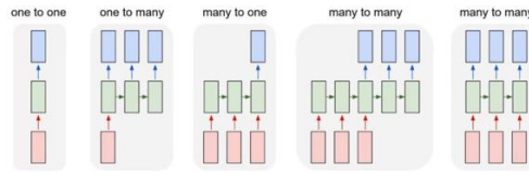
Şekil 5. LSTM modelleri
