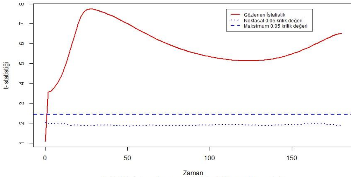
Şekil 5. Tedavi grupları arasındaki farka ilişkin permütasyon testi
